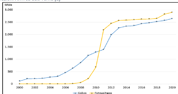
Figura 23 - Storico potenza installata da fonte rinnovabile eolica e fotovoltaica
