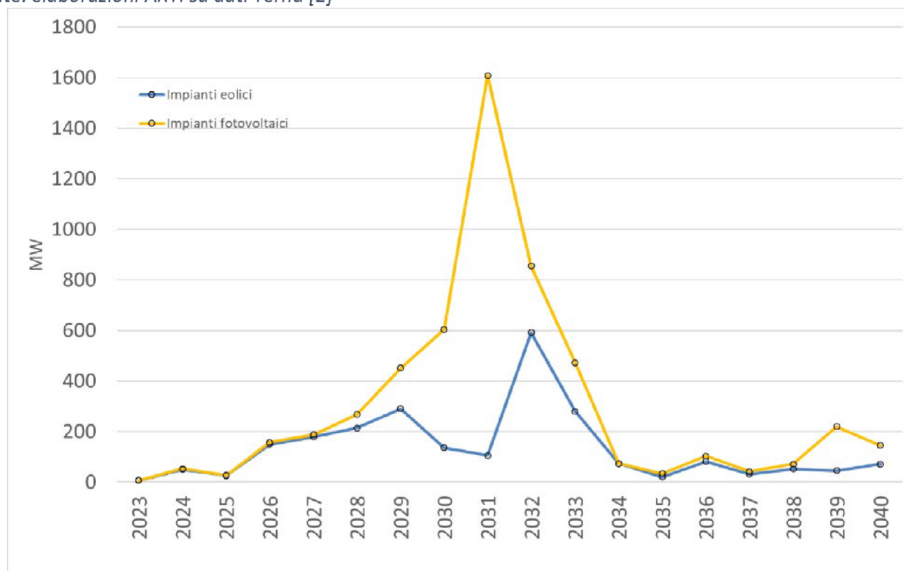
Figura 24 - Stima della potenza installata da fonte rinnovabile a fine vita utile fino al 2040
