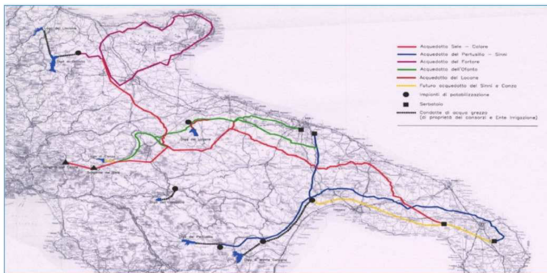
Figura 26 schema dei vettori di approvvigionamento della Regione Puglia.
