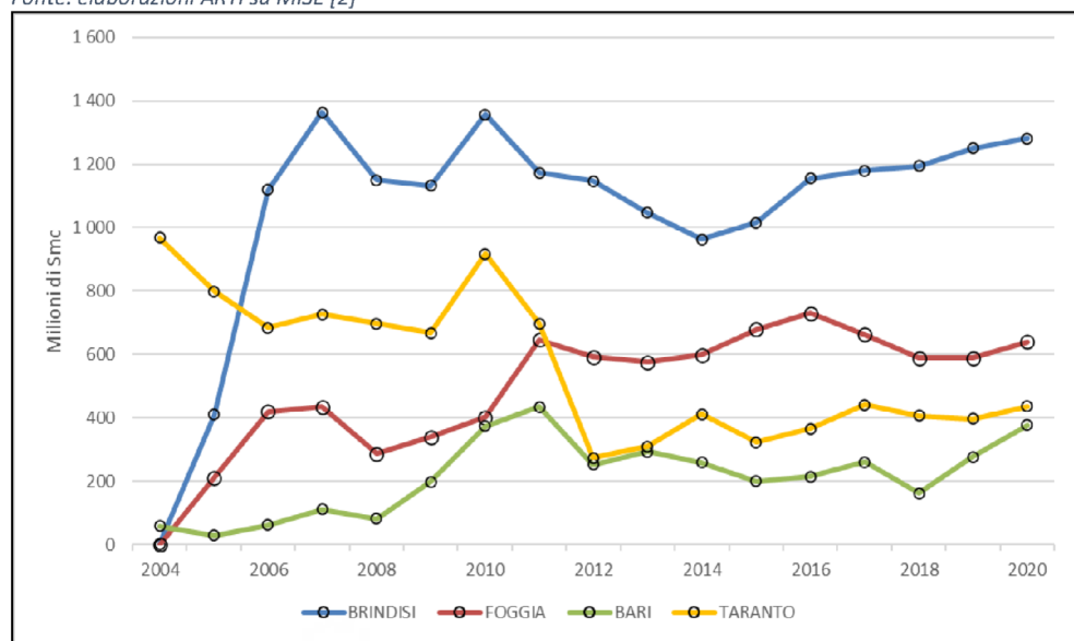
Figura 47 – Storico gas consumato per produzione elettrica per Provincia
