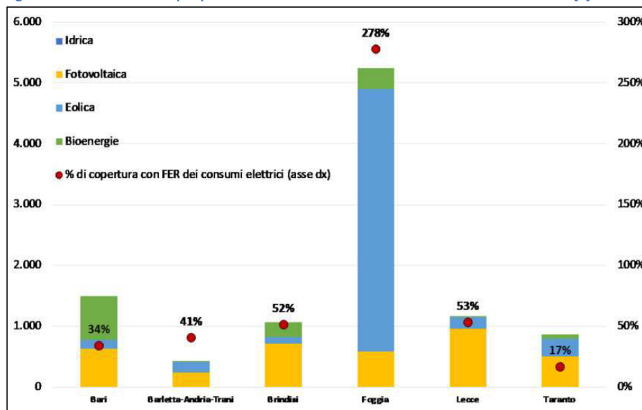
Figura 38 – Produzione FER per provincia anno 2019. Fonte: elaborazioni ARTI su dati Terna [2]
