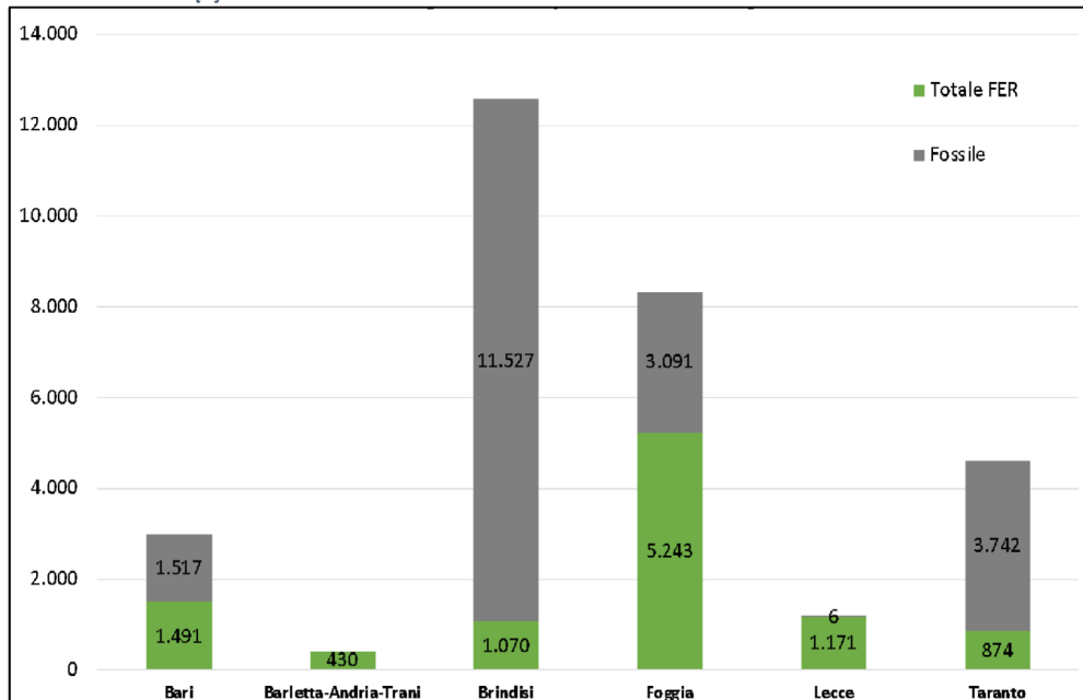
Figura 7 - Distribuzione per province della produzione di energia elettrica . Fonte: elaborazioni ARTI su dati Terna [2]
