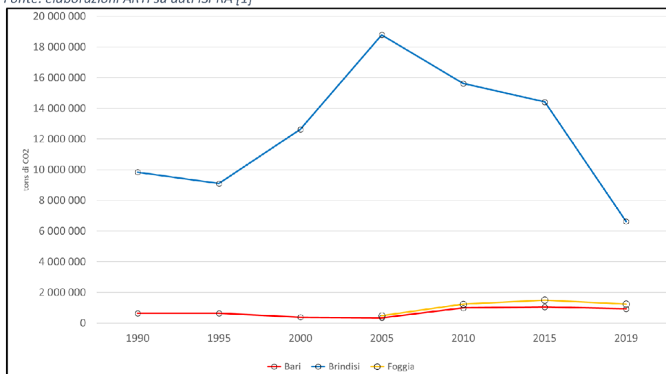
Figura 55 - Emissioni di CO 2 degli impianti energetici pubblici per provincia Fonte: elaborazioni ARTI su dati ISPRA [1]
