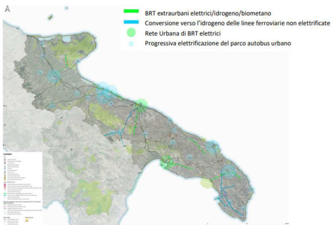
Figura 5 : Gli interventi di decarbonizzazione previsti dal PA PRT 2021/2030
