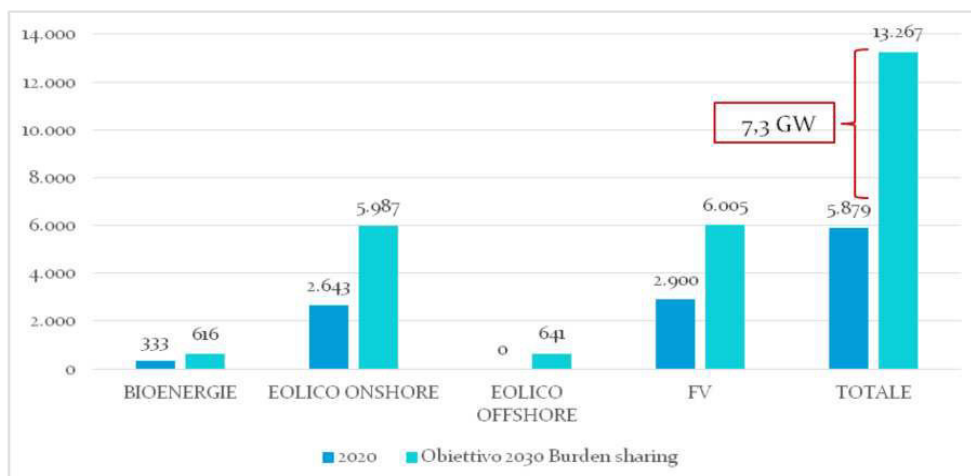
Figura 1: Confronto tra dati 2020 e obiettivo 2030 in termini di potenza efficiente lorda
