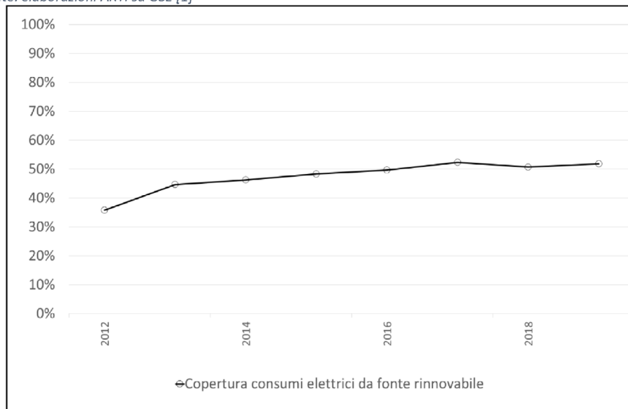
Figura 40 – Copertura dei consumi elettrici regionali mediante fonti rinnovabili (FER-E)
