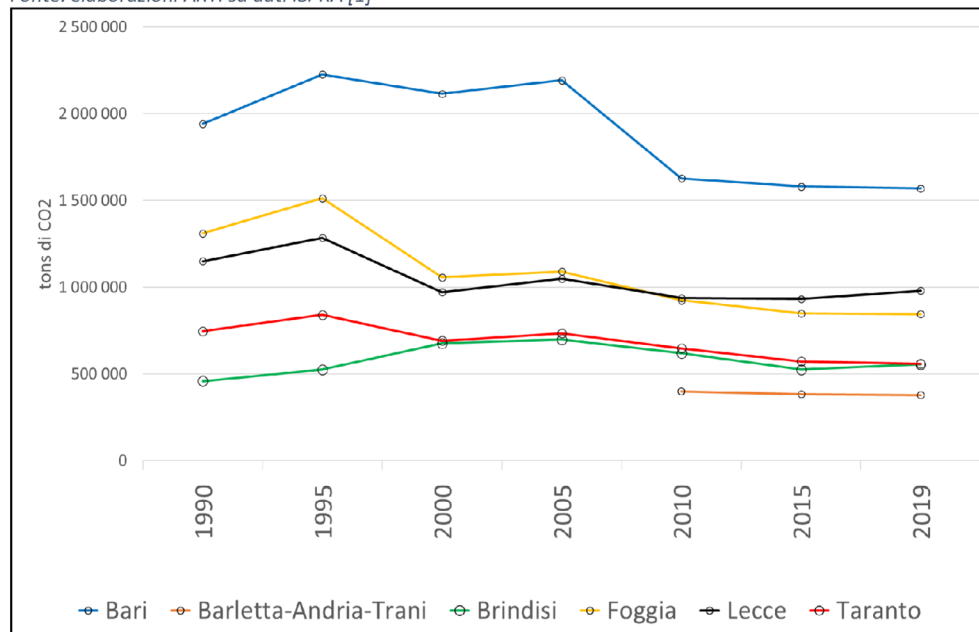
Figura 62 - Storico emissioni CO2 da trasporti per Provincia
