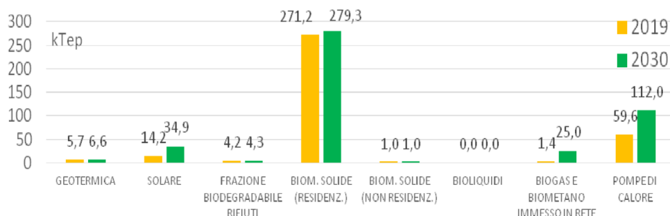
Figura 86 – Scenario Obiettivo: produzione termica da rinnovabili suddivisa per fonte.
