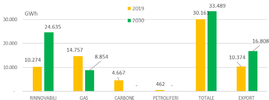
Figura 83 – Scenario Obiettivo, mix della produzione di energia elettrica al 2019 e al 2030.
