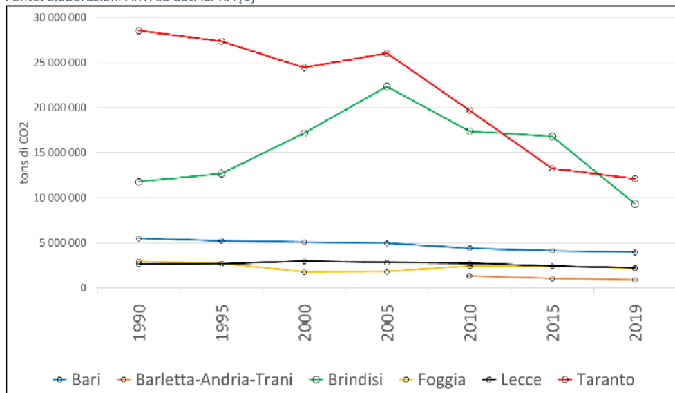
Figura 51 - Andamento storico delle emissioni di CO 2 per Provincia
