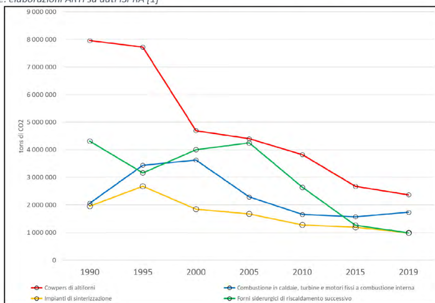
Figura 53 - Storico delle emissioni di CO 2 del macrosettore "Combustione - Industria" Fonte: elaborazioni ARTI su dati ISPRA [1]
