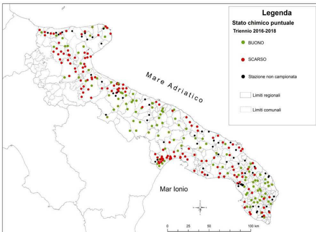
Figura 23 Stato chimico puntuale per i Corpi Idrici Sotterranei nell'intero territorio regionale–Triennio 2016-2018.Fonte Arpa Puglia.
