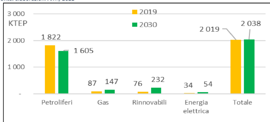
Figura 69 – Scenario “Continuità” – Consumi nei trasporti per fonte al 2030 rispetto al 2019.
