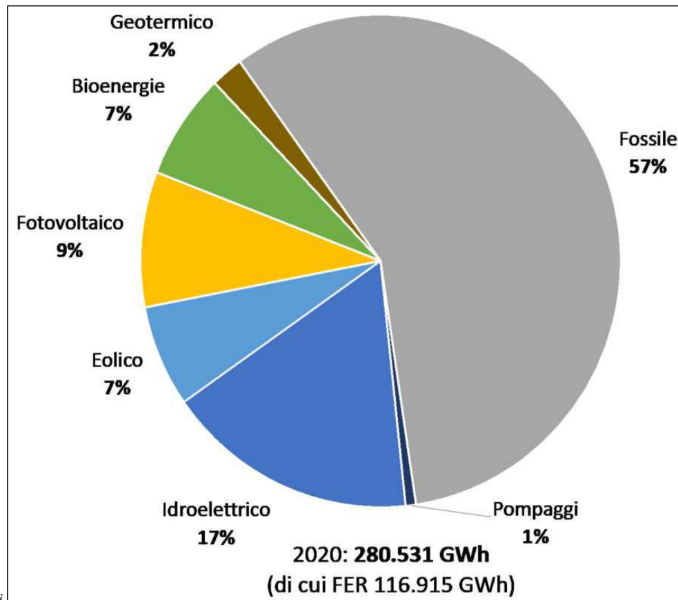
Figura 36 – Produzione di energia elettrica in Italia per fonte Fonte: elaborazioni ARTI su dati TERNA [1e2]
