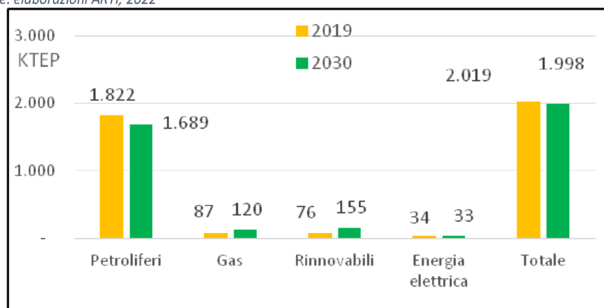
Figura 65 – Scenario inazione – Consumi del settore trasporti per fonte al 2030 rispetto al 2019.
