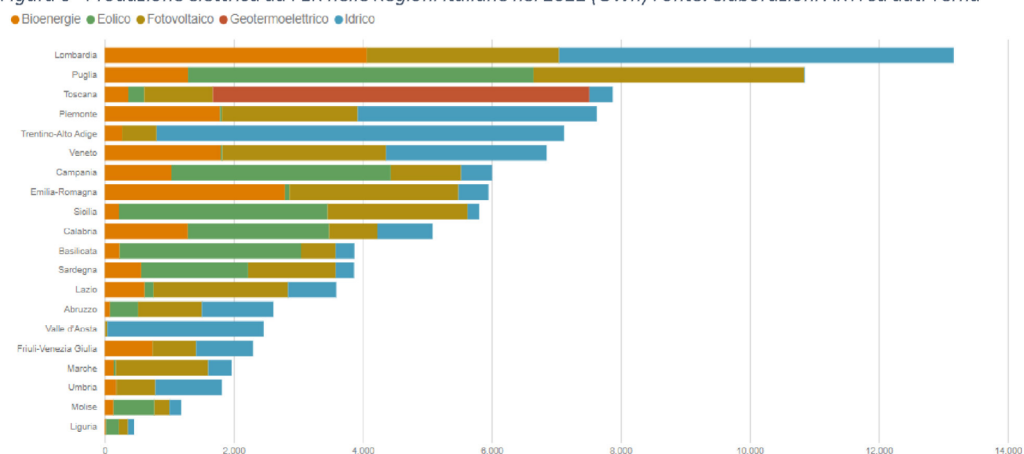
Figura 6 - Produzione elettrica da FER nelle Regioni italiane nel 2022 (GWh) Fonte: elaborazioni ARTI su dati Terna
