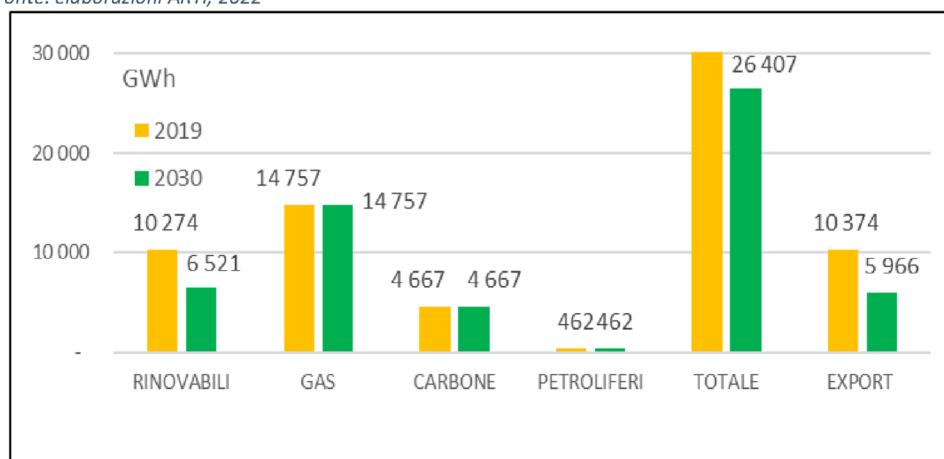
Figura 63 – Scenario inazione – Mix della produzione di energia elettrica al 2019 e al 2030.
