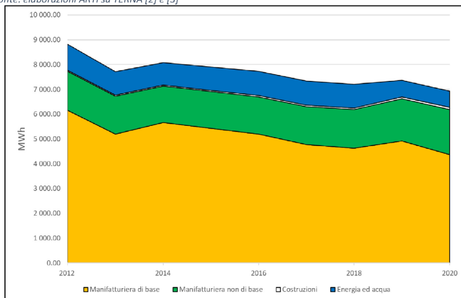
Figura 32 – Ripartizione dei consumi di energia elettrica del settore industriale
