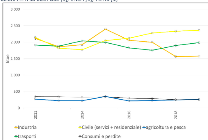
Figura 30 – Consumi finali lordi per settore
