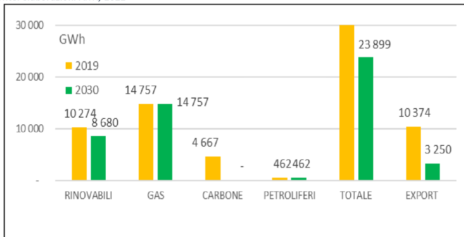
Figura 67 – Scenario “Continuità” – Mix della produzione di energia elettrica al 2019 e al 2030. Fonte: elaborazioni ARTI, 2022
