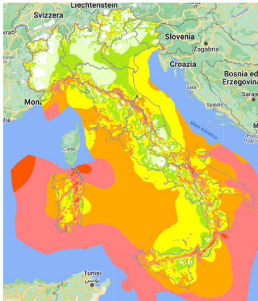
Figura 74 – Velocità media vento a 150 metri sul livello del mare.
