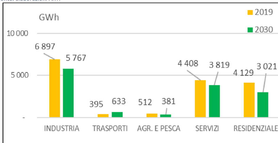
Figura 84 – Scenario Obiettivo: consumi elettrici per settore al 2030 rispetto al 2019.
