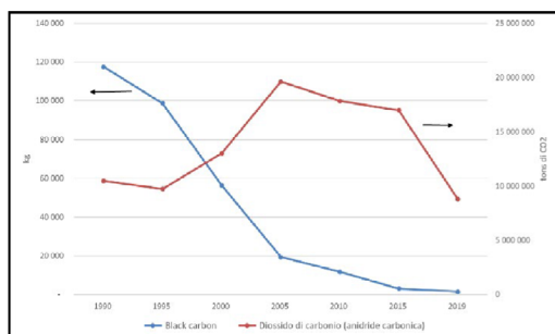
Figura 58 – Produzione Energia - Storico emissioni black carbon
