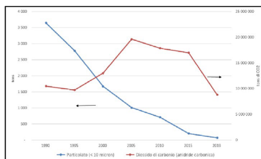
Figura 61 - Produzione Energia - Storico emissioni di PM10
