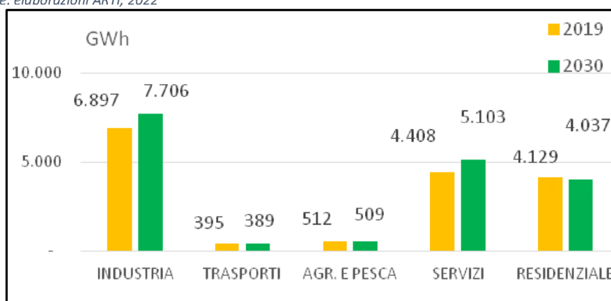
Figura 64 – Scenario inazione – Consumi elettrici per settore al 2030 rispetto al 2019.
