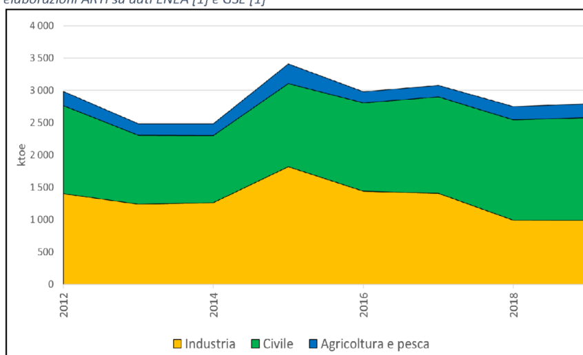
Figura 38 – Consumi termici per settore
