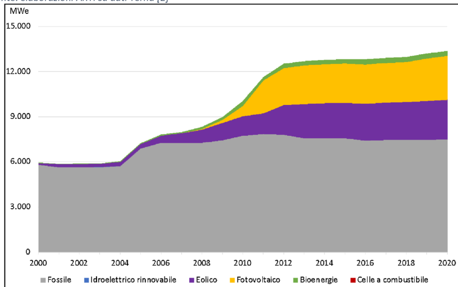
Figura 21 - Evoluzione della potenza di generazione elettrica installata in Puglia
