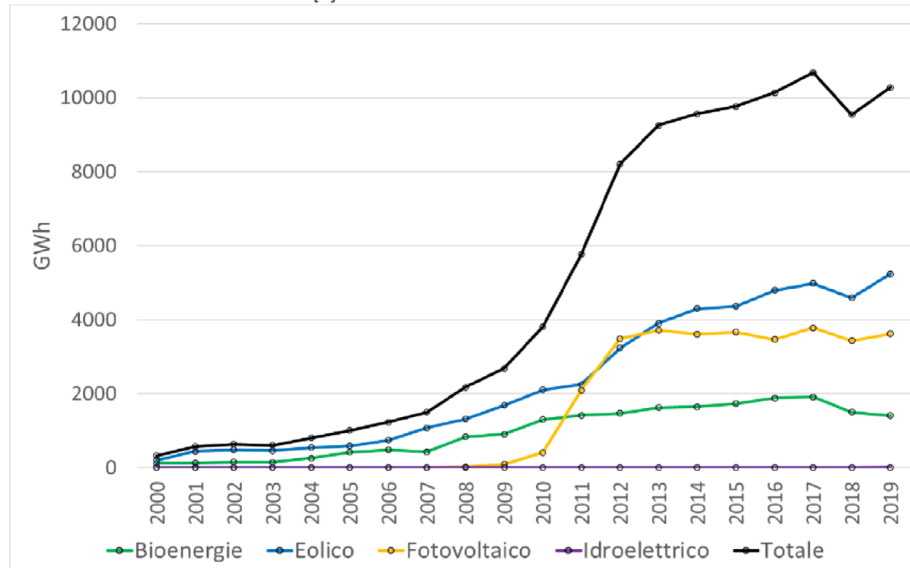
Figura 22 - Storico produzione da fonte rinnovabile
