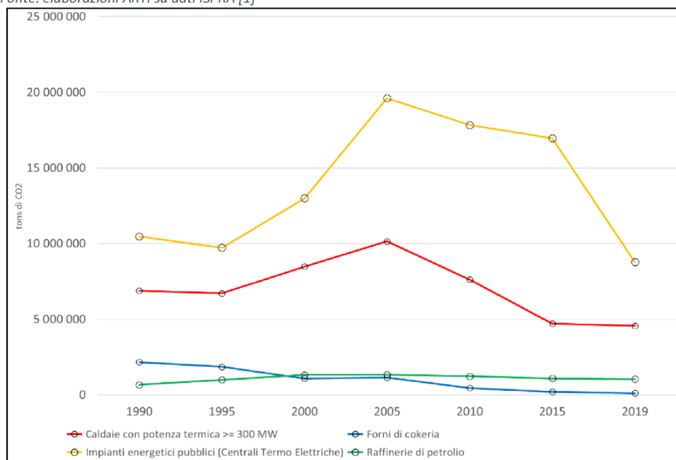
Figura 54 - Storico delle emissioni di CO 2 del macrosettore "Combustione - Energia e industria di trasformazione" Fonte: elaborazioni ARTI su dati ISPRA [1]
