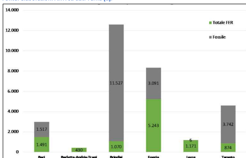
Figura 37 – distribuzione per province della produzione di energia elettrica.
