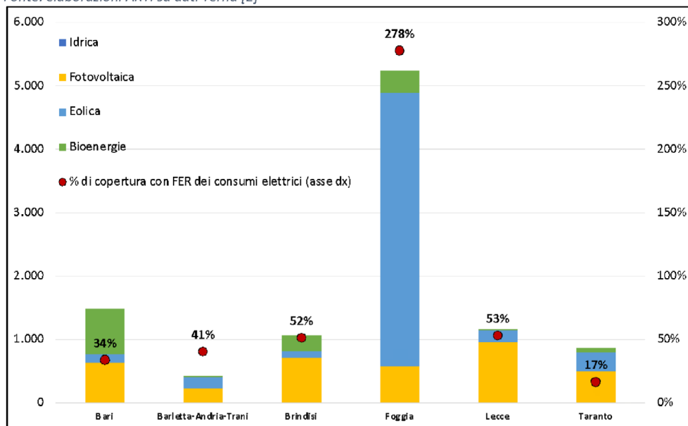
Figura 8 - Produzione FER per provincia anno 2019.
