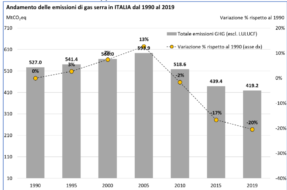
Figura 50 – Storico emissioni gas serra in Italia dal 1990 al 2019
