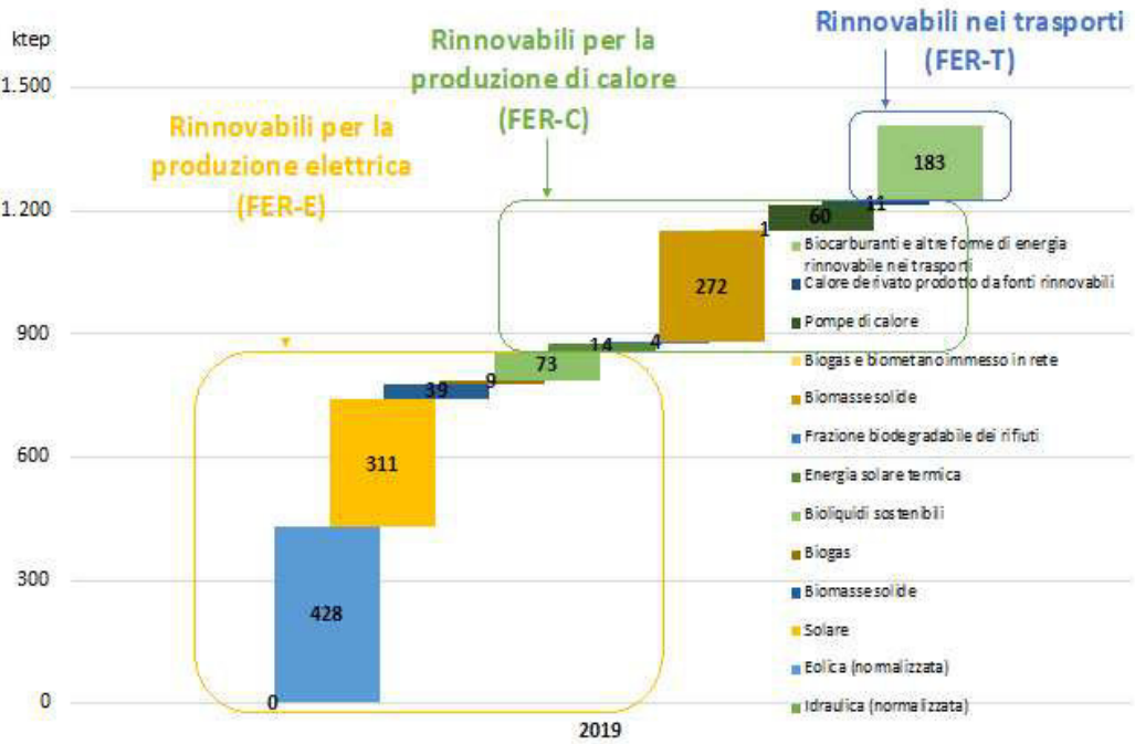
Figura 47 – Consumi energetici da fonti rinnovabili in Puglia nel 2019. Fonte: elaborazioni ARTI su dati Enea [1], Terna [1 e 2], GSE [1] ed Eurostat [1 e 2]
