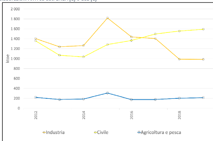
Figura 37 – Consumi finali lordi di calore per settore
